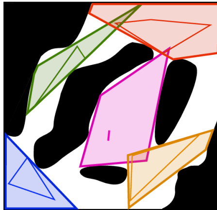
Hình 4.12: Lấp đầy thành Đa diện
