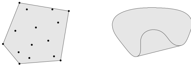
Hình 2.2: Bao lồi của một tập hợp điểm (phần được tô đậm).boyd2004
