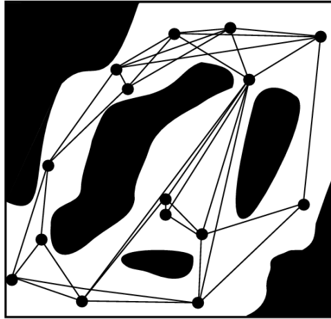
Hình 4.9: Lấy mẫu & Xây dựng Đồ thị Khả kiến (Visibility Graphs)
