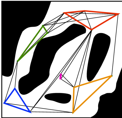
Hình 4.10: Tìm Lớp phủ Clique
