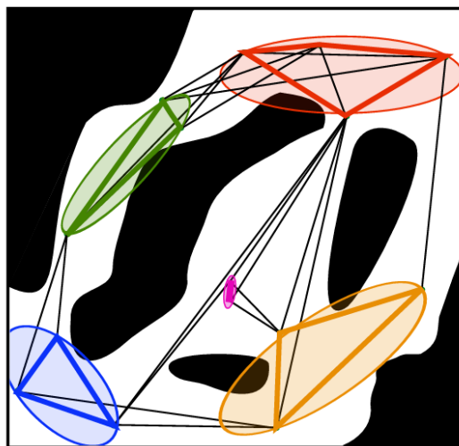
Hình 4.11: Khởi tạo Ellipsoid
